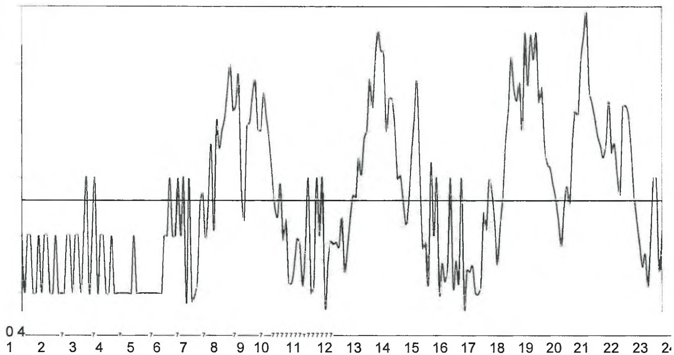
График фактической подпитки тепловых сетей котельной № 4 на 02.11.2021г.
