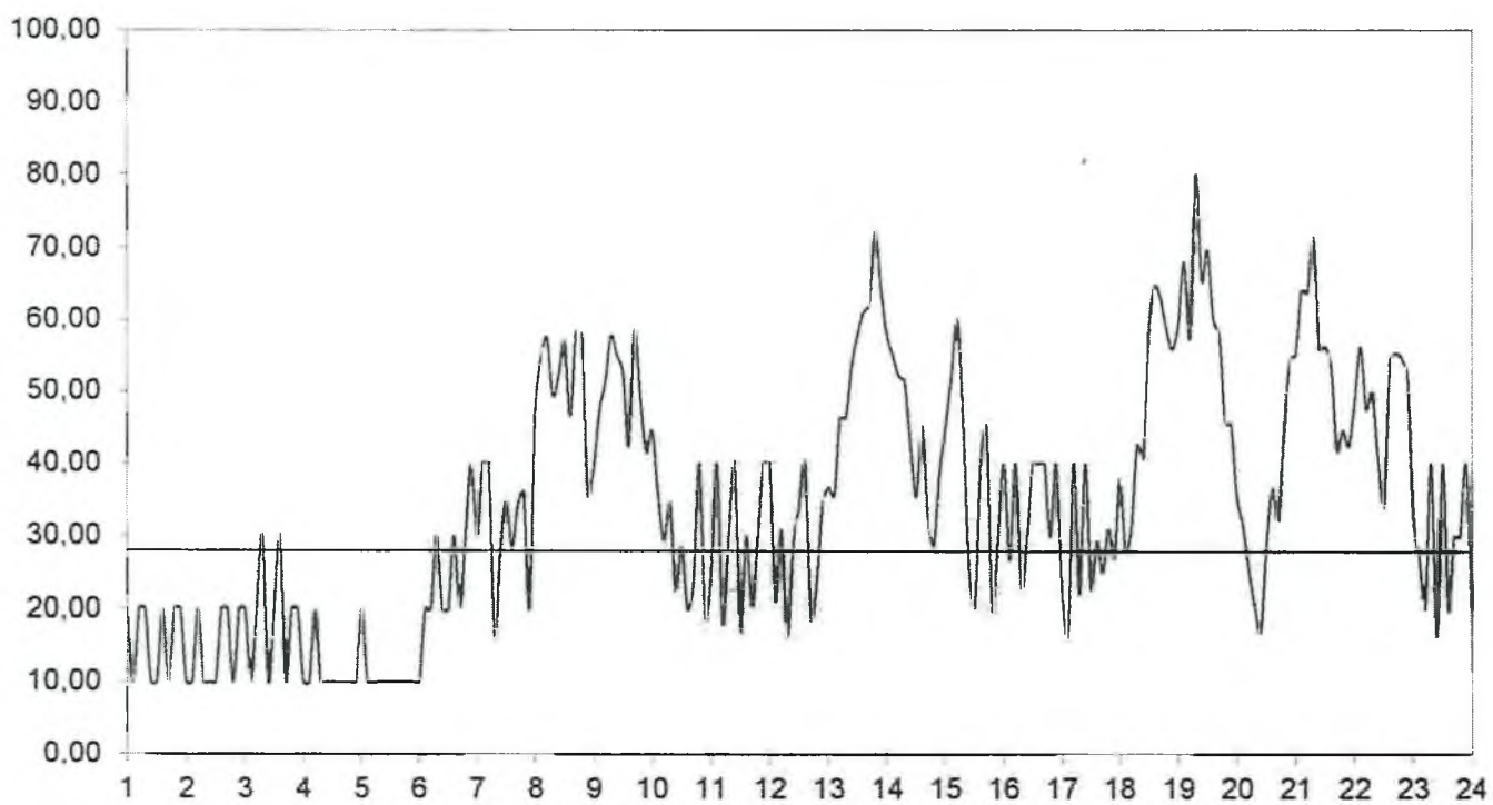
График фактической подпитки тепловых сетей котельной № 4 на 02.11.2021г.
